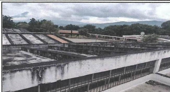
Foto 2: área dañada en loza, aplicación de impermeabilizante
