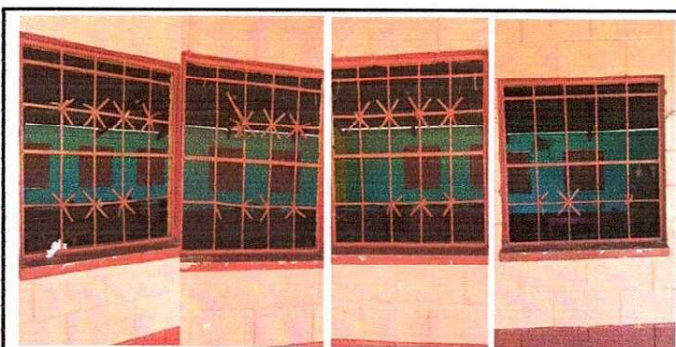
Foto 5: Se observa que la estructura de metal del balcon se encuentra en mal estado por lo que se requiere su sustitución.
