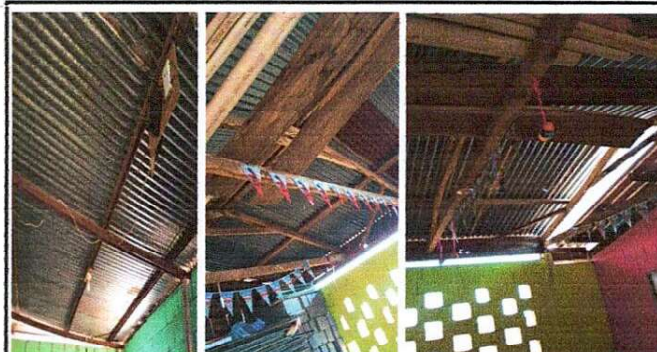
Foto 2: se observa que la estructura portante de metal y madera se encuentra en mal estado por lo que requiere sustitución.
