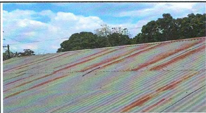
FOTO 1: Se observa el deterioro físico de la lámina por lo que es necesario el mantenimiento de la misma.
