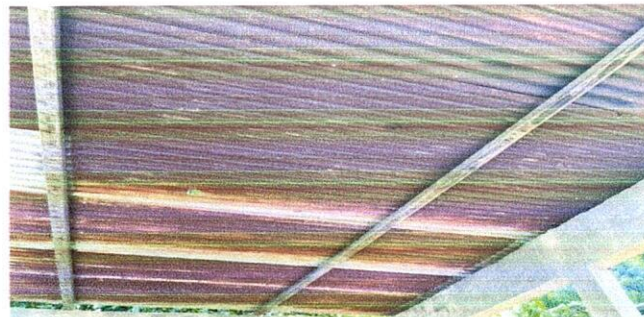
Foto 6: Las laminas presentan corrosion, es necesario cambiarlas
