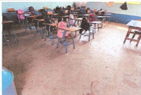
Foto 7: Se observa que el módulo de aulas 3 no cuenta con piso cerámico, por lo que este deberá ser suministrado.
