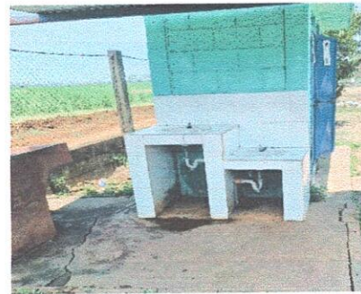
Foto 4: Se observa que la torta de concreto en los lavamanos se encuentra ya muy dañada.
