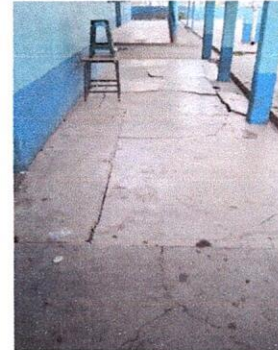
Foto 8: Se observa que el piso del corredor del modulo de aulas esta dañado, por lo debiera ser reparado.
