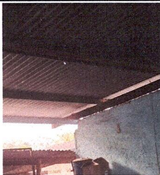
Foto 5: Se observan las laminas picadas del modulo de aulas, deben ser reemplazadas por lamina troquelada.
