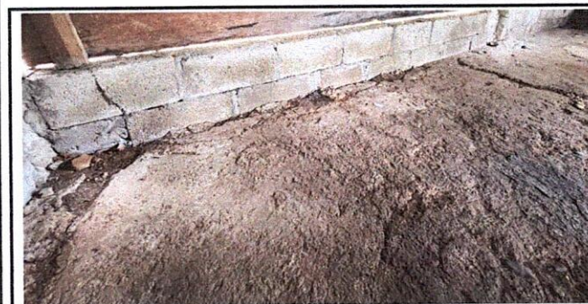
FOTO 5: Sustrucción y fundición de todo el piso de torta de cemento.
