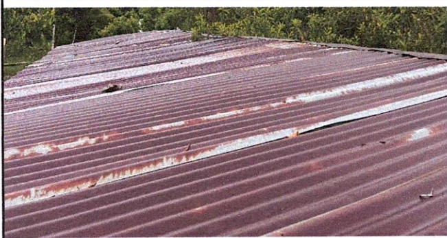
FOTO 1: Sustrucción de lámina por lámina troquelada aluzinc cal 26" incluye capotes y elementos de fijación
