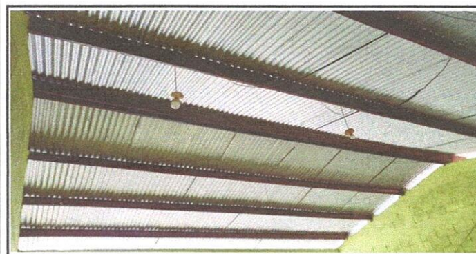
Foto 4: MODULO 2.Sustitución de lámina por lámina troquelada calibre 26
