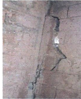
Foto 2: Estructura de Soporte
