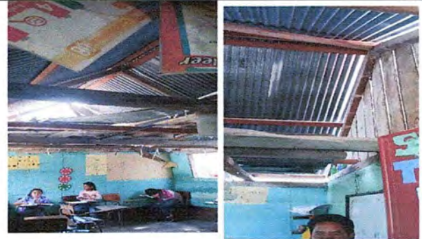
FOTO 2. MODULO 1: Sustrucion de estructura de soporte de madera por metal.
