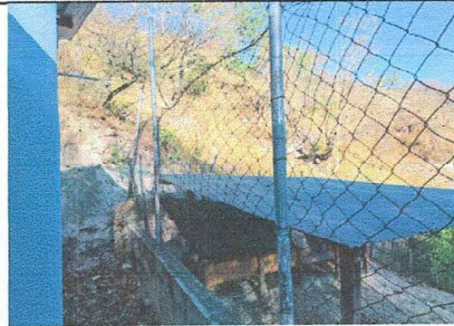
Foto 4, Muro perimetral: Reparación de tubo hg y malla galvanizada
