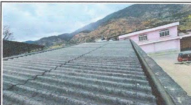
MODULO 1 sustitucion de lamina por lamina troquelada aluzinc calibre 26
