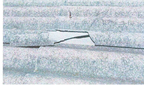
Foto 1: MODULO 1 Sustitución de laminas por lamina troquelada aluzinc calibre 26
