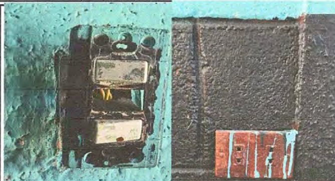
Foto 8: MODULO 1 Sustitución de Apagador y Tomacorrientes Dobles
