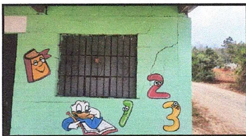
Foto 5: Módulo 1: Reparación de muro (pared) de aula
