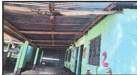
Foto 2: Módulo 1: Sustitución de estructura de soporte de madera por metal
