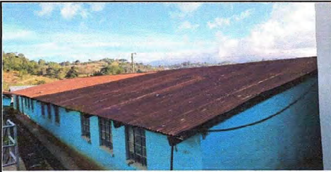
Foto 1: Modulo 1: Situación de lámina a lámiona troquelada calibre 26
