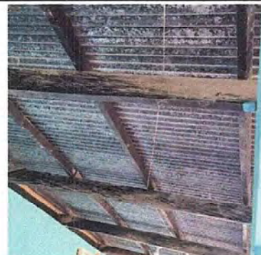
Foto 4: Modulo 1: Situación de vigas de madera a metal
