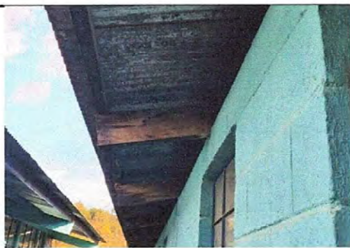
Foto 5: Modulo 1: Situación de vigas de madera a metal
