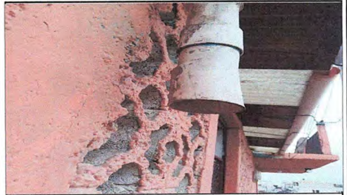
FOTO 4: MODULO 1: Sustitución de tubería PVC línea principal aguas pluviales
