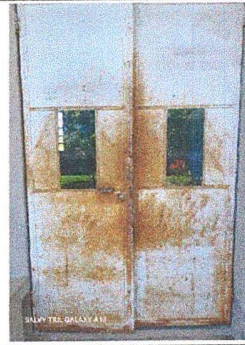
Foto 2: Módulo I: Mantenimiento a estructura de puertas (lijado, cambio de tubo, cepillado, sujeciones, aplicación de pintura)
