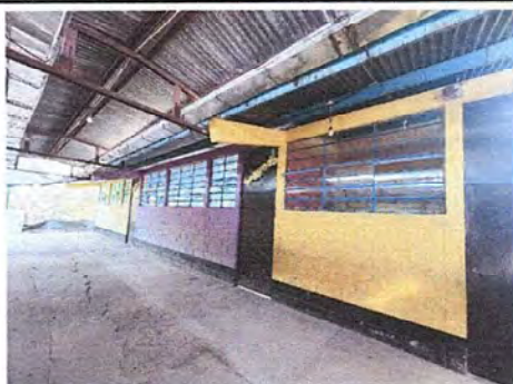
Foto 3: Modulo#2, Mantenimiento a estructura de Puerta y suministro e Instalación de Balcones de Metal.
