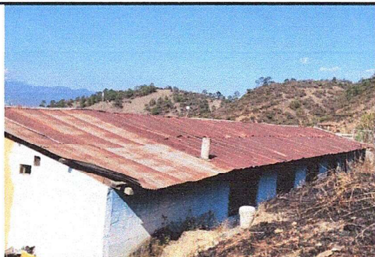
Foto 1: MODULO 1: Sustitución de lámina, por lámina troquelada aluzinc calibre 26
