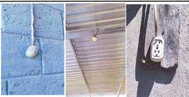
Foto 5: MODULO 2: Instalación de unidades luz (incluye interruptor, ducto y cable eléctrico)
