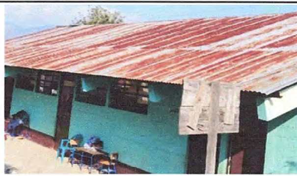
Foto 4: MODULO 2: Sustitución de lámina, por lámina troquelada aluzinc calibre 26
