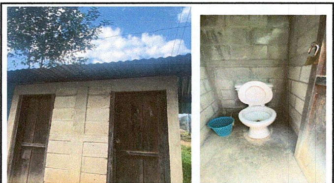
Foto 4: Módulo 4, Sustitución de lámina, por lámina troquelada aluzinc calibre 26 y sustitución de puertas de metal y sustitución de Inodoros.
