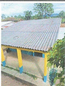
Foto 1. Modulo1: Sustrucion de lamina por lamina troquelada calibre 26
