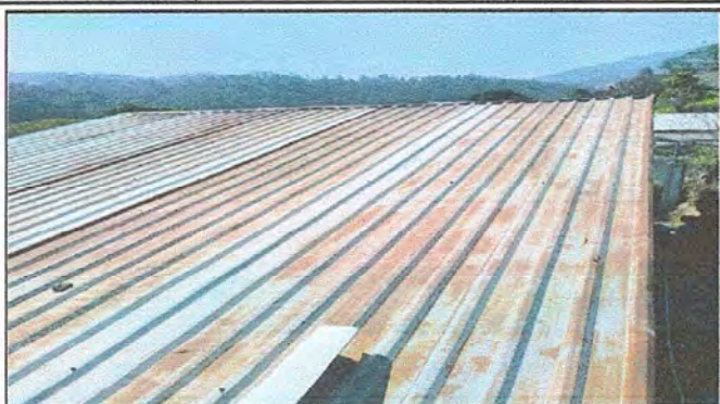
Foto 1: Módulo 1: sustitución de lámina troquelada aluzinc calibre 26
