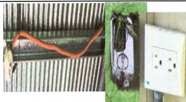
MODULO 1: FOTO 4 SUSTITUCIÓN DE UNIDAD DE LUZ (INTERRUPTOR DUCTO CABLE ELECTRICO Y FOCOS)
