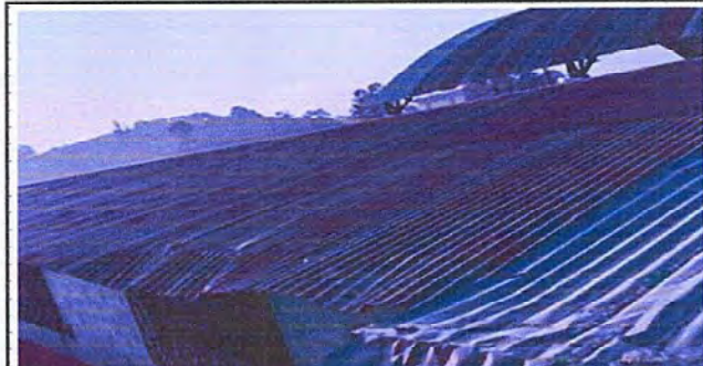
Foto 4: Módulo 1. Sustitución de lamina por lamina troquelada de aluzinc calibre 26.
