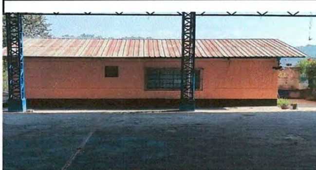
Módulo 4: Reparación debajada de agua pluvial, tubo, PVC 3. FOTO 20
