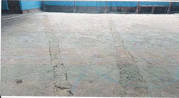
Foto 1: Reparación de Plancha de concreto de patio
