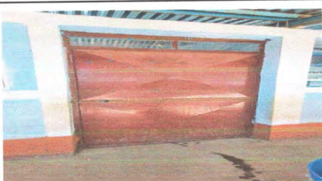
Foto 3: Modulo 3 Mantenimiento a estructura puerta de metal (lijado, cepillado, sujeciones, aplicación de pintura)
