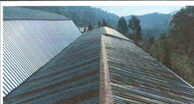
Foto 2: Modulo 1. Cambio de capotes de las laminas por capotes calibre 26.
