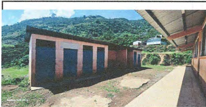
Foto 7: BAÑOS "B". Mantenimiento a estructura de puerta (lijado, cambio de tubo, cepillado, sujeciones, aplicación de pintura).
