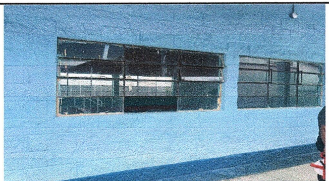
FOTO 5: MODULO 3: Sustitución de ventanas de metal por metal mas vidrio, Sustitución de ventanas de metal por metal mas vidrio, pintura exterior, Suministro e instalación de balcon de metal.
