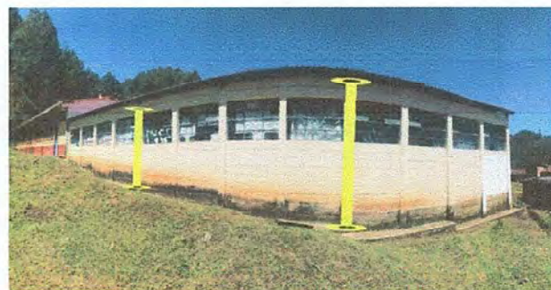
Foto 2: Suministro e instalación de balcones de hierro en ventanas Módulo 1
