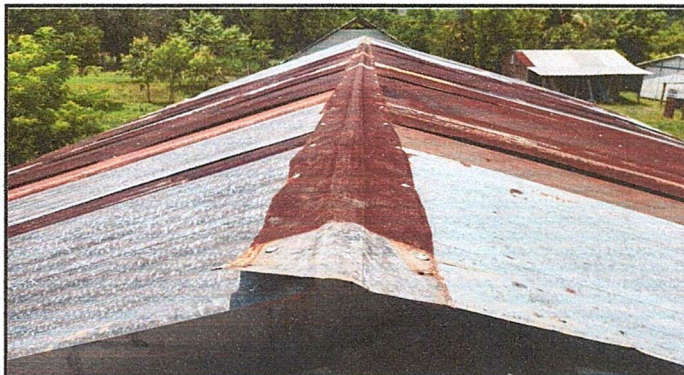
Foto 2. Módulo 4: Sustitución de capote para lámina troquelada
