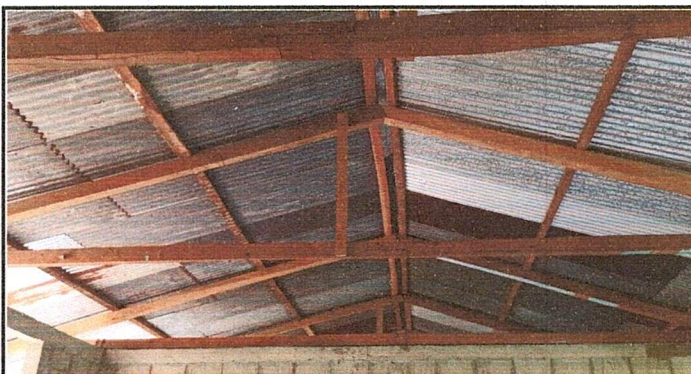
Foto 3. Módulo 4: Sustitución de estructura de soporte de madera, por metal
