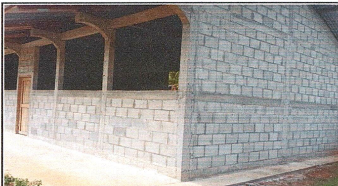
Foto 8. Módulo 4: Repello en muro
