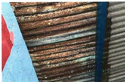
Foto1. Módulo 2: Sustitución de lámina ondulada calibre 26 y elementos de fijación.
