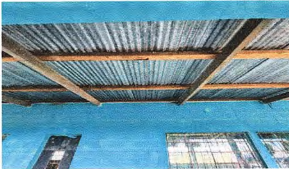
Foto 3: MODULO 1 .SUSTITUCION DE ESTRUCTURA DE SOPORTE DE MADERA POR METAL
