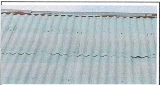
Foto 5: Modulo 2: SUSTITUCION DE CAPOTE DE LAMINA PARA LAMINA TROQUELADA
