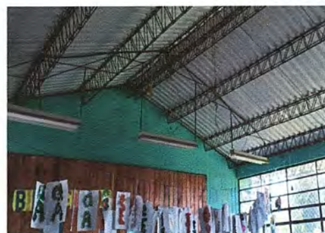
Foto 6: MODULO 1: SUSTITUCIÓN DE PLAFONERAS Y SUSTITUCIÓN DE FOCOS AHORRADORES
