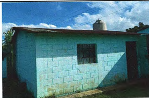
Foto 8: MODULO 4: Sustitución de lamina por lamina troquelada, sustitución de capote, sustitución de elementos de fijación.
