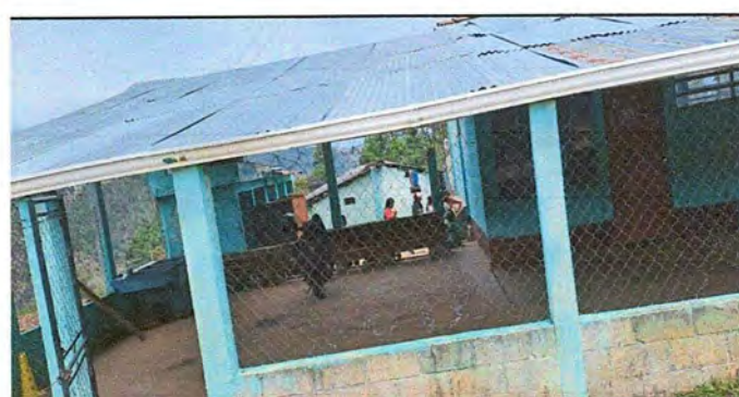
FOTO 6, MODULO 3: sustitucion de laminas troqueladas calibre 26 y sustitucion de sopórte de metal a metal
