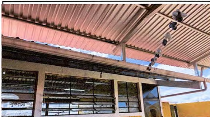
FOTO 14: MODULO 2: SUSTITUCIÓN DE CANAL, SUSTITUCIÓN DE PESCANTE Y SUSTITUCIÓN DE BAJADA DE AGUA PLUVIAL PVC DE 3".
