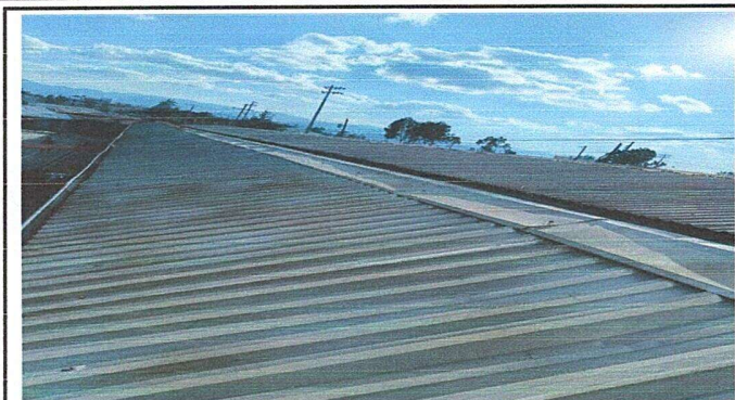
Foto 1: Módulo 1. Sustitución de lámina, por lámina troquelada aluzinc calibre 26.
