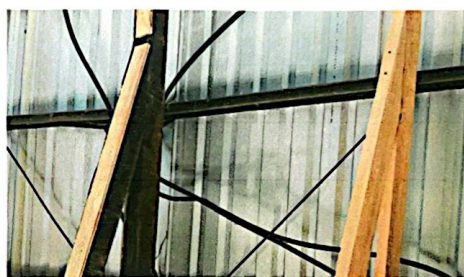
Foto 4: Sustitución del cableado eléctrico Calibre 10 AWG
