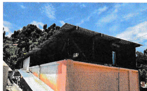
No.6 Sustitución de postes de madera a metal galvanizado en aulas de segundo nivel en módulo No. 3
