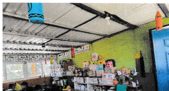
No.4 Sustitución de estructura de soporte de madera por estructura de Metal galvanizado en aulas segundo nivel del modulo No. 3
