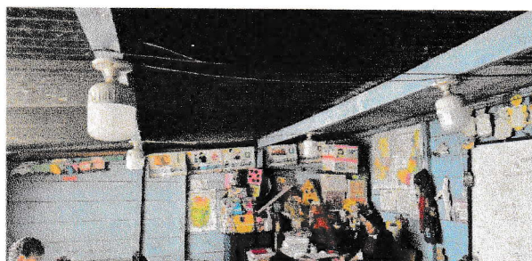
No.3 Sustitucion de cableado electrico No. 10 AWG en aulas de segundo nivel del modulo No. 3
