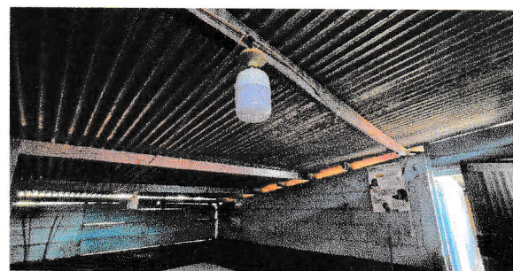
No.4 Sustitución de estructura de soporte de madera por estructura de Metal galvanizado en aulas segundo nivel del modulo No. 3
