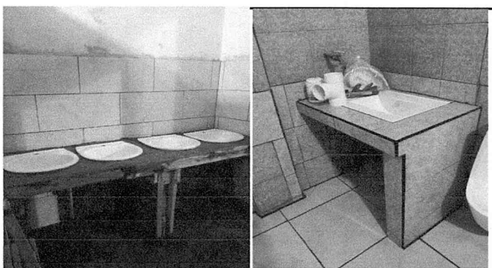
Sustitucion de lavamanos de niños y niñas
