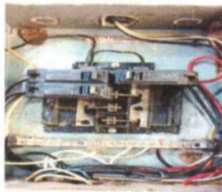
FOTO 9. REPARACION CABLEADO ELECTRICO CAL.12AWG AULAS
